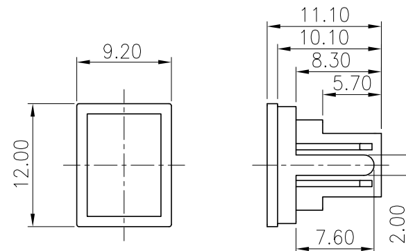
防尘帽图示
