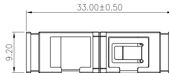
加带防尘帽图示
