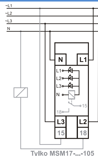
Tylko MSM17-...-105
