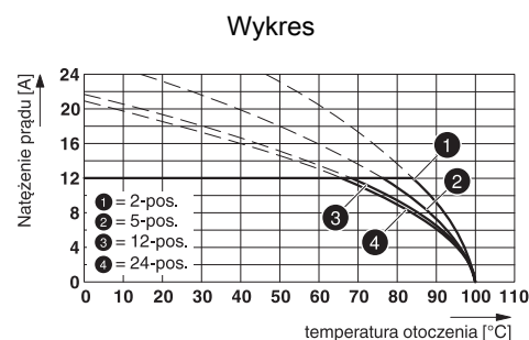
Typ: MSTB 2,5/...-ST-5,08 z CCVA 2,5/...-G-5,08 P26THR
