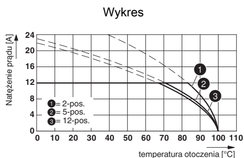
Typ: MSTB 2,5/...-ST-5,08 z CC 2,5/...-G-5,08 P26THR
