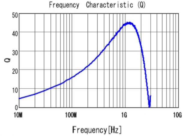
■ LQG18HN15NJ00 Q
