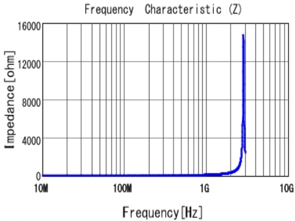
■ LQG18HN15NJ00 |Z|
