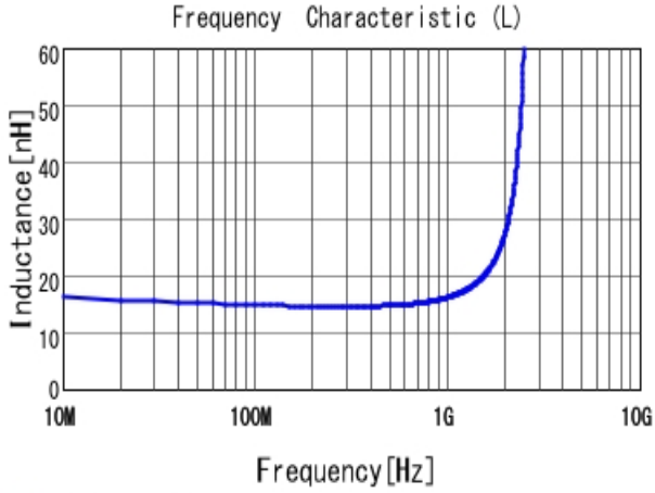
■ LQG18HN15NJ00 L
